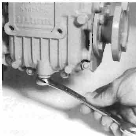
Lösen der Abtaßschraube. Dépose du bouchon de vidange.
