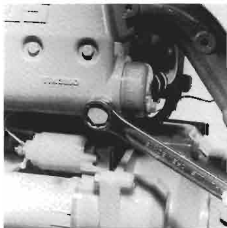
Retirar el tapón de vaciado. Rimozione dei tappi di scarico.
