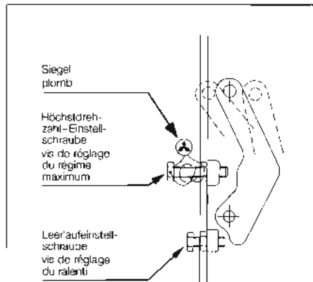
Einstellen der Leerlaufdrehzahl Réglage du régime au ralenti
