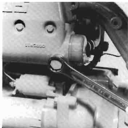
Retirar el tapón de desagüe. Rimozione del tappo di scarico.
