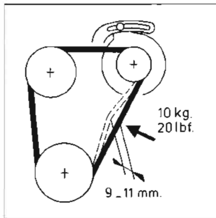
Controlar la tensión. Controllo della tensione.
