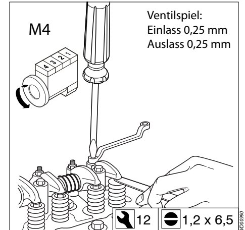
48 Ventilspiel einstellen
