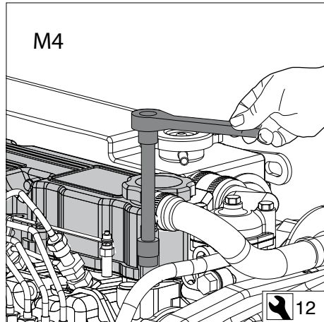
46 Ventildeckel entfernen
