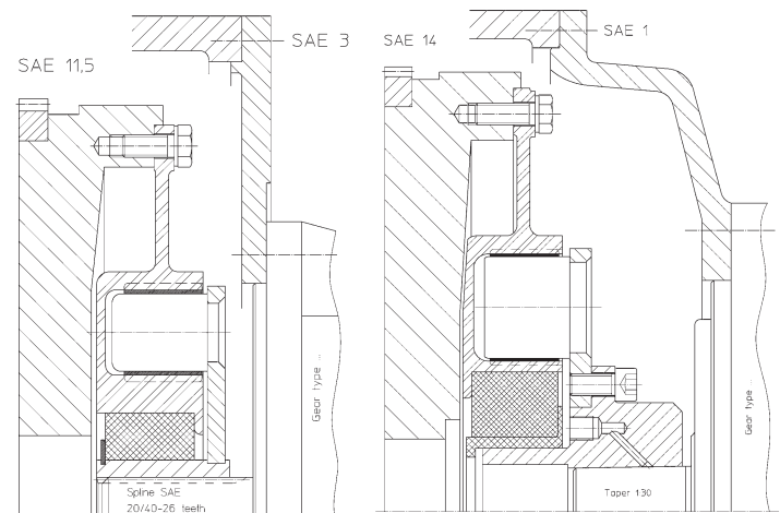
Gear with input shaft / Getriebe mit verzahnter Antriebswelle
