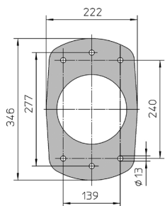
CENTA TB 5
