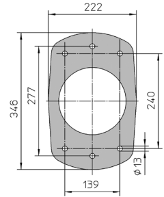
CENTA TB 5
