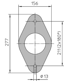
CENTA TB 3
