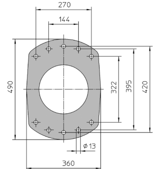
CENTA TB 6
